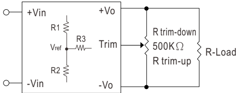
图3. Trim配接
