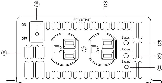
圖3.1 前面板示意圖(型式A)
