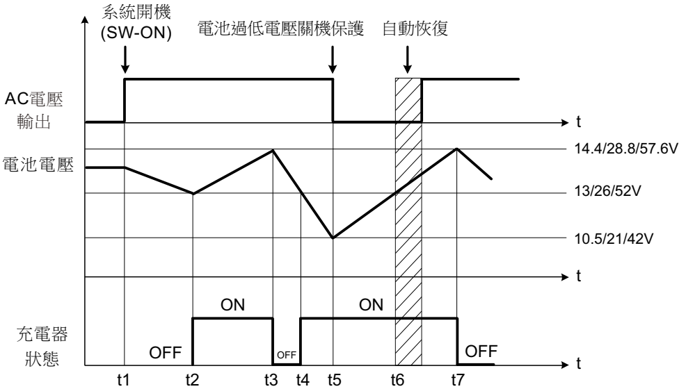
圖5.1 程序控制圖
